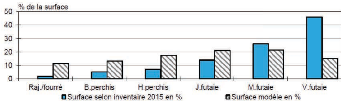
figure 4: Répartition des stades de développement dans les forêts du triage (% de la surface totale)
