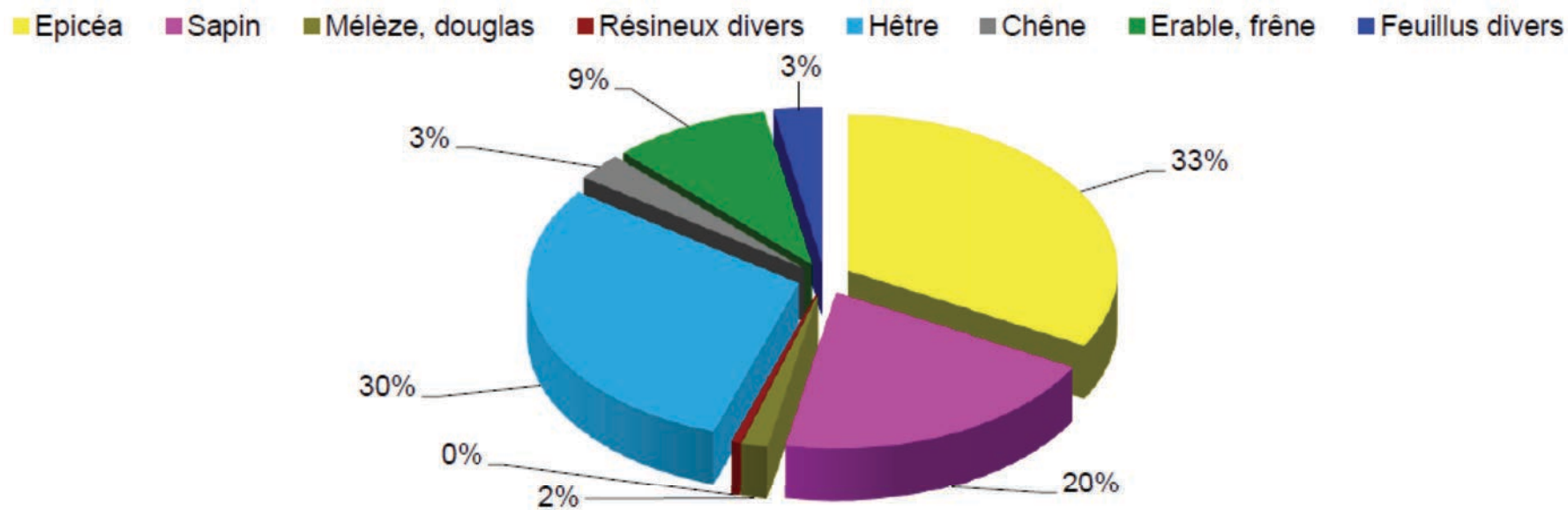
figure 5: Mélange des essences dans les forêts du triage (% du volume)
